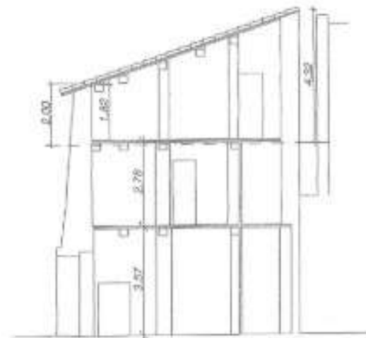
Sezione B-B
